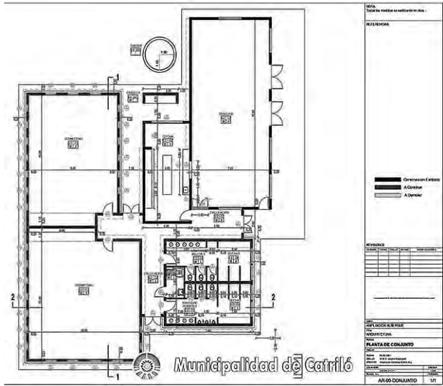
Plano del Albergue Municipal de Catriló.
